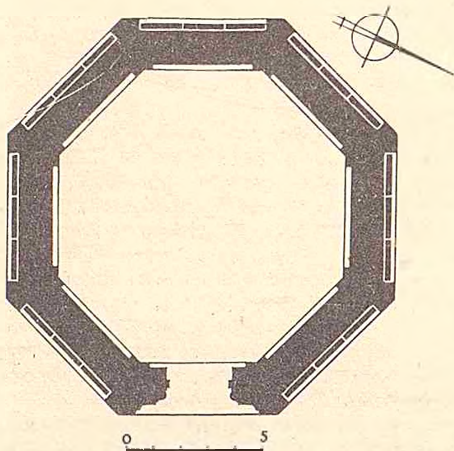
Нахчыван. Јусиф Күсејир оглу түрбәсини планы.
