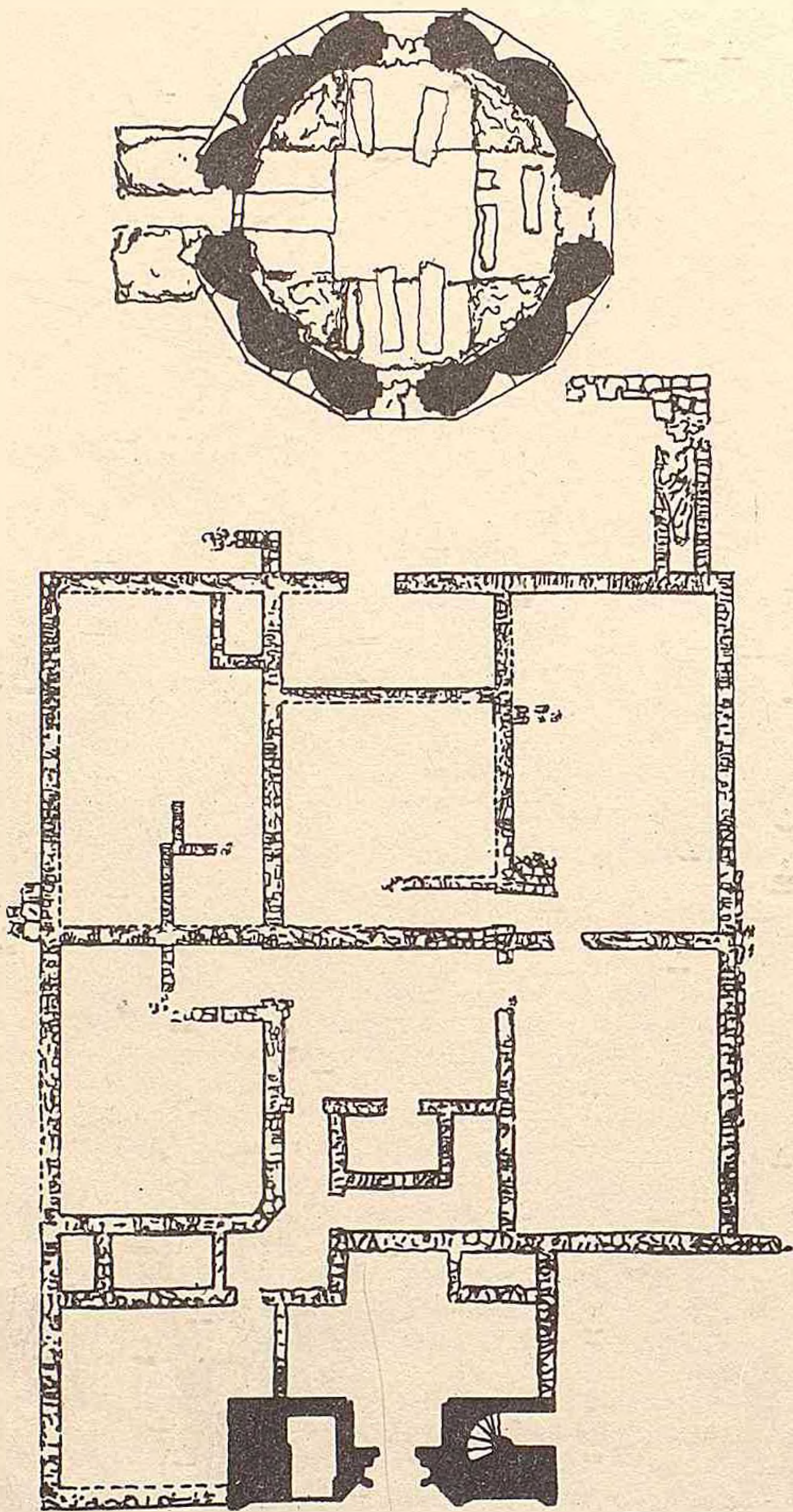
Гарабағлар түрбәсинин үмуми планы.
