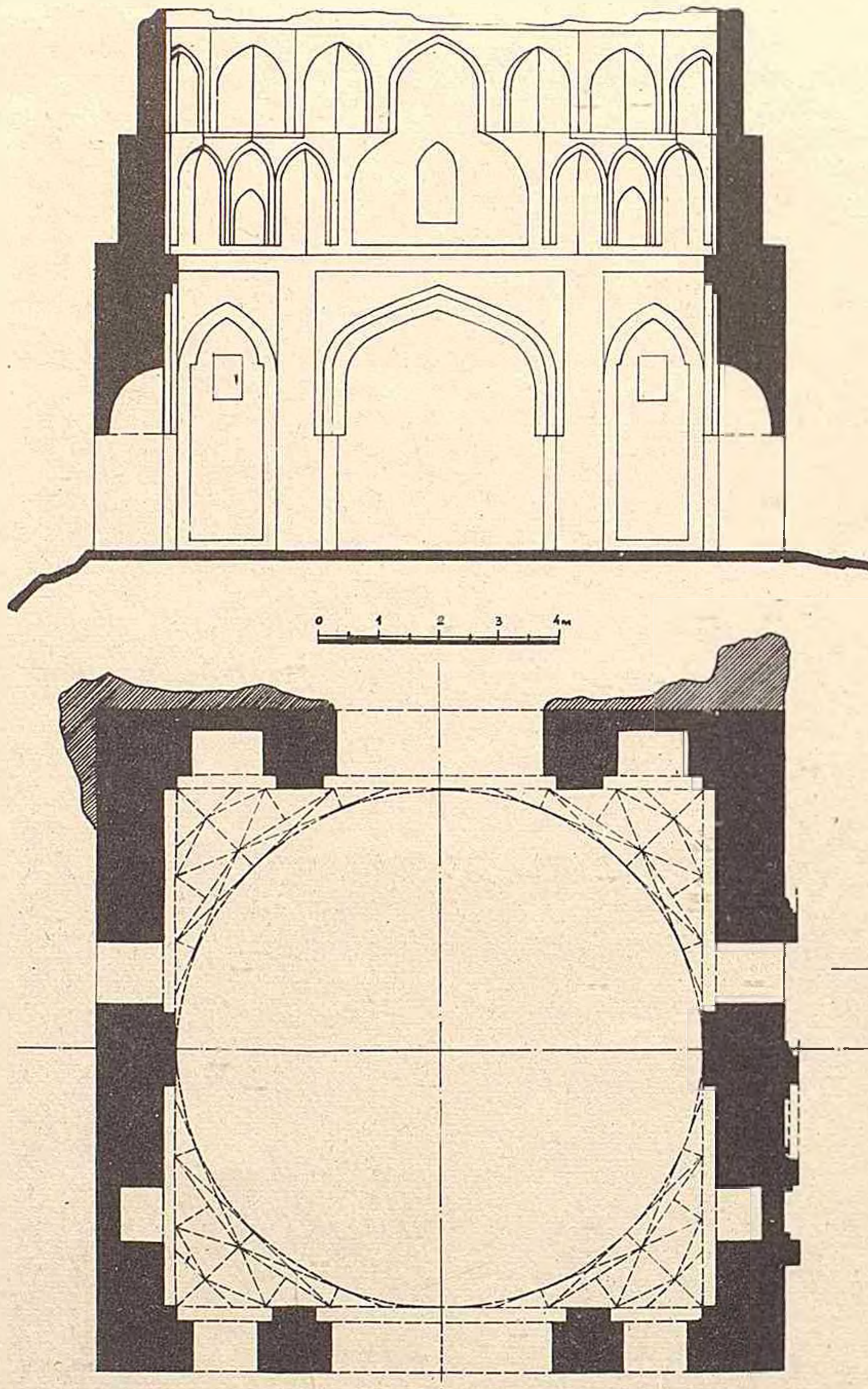
Кирпа кэнди. Түрбәнин планы.
