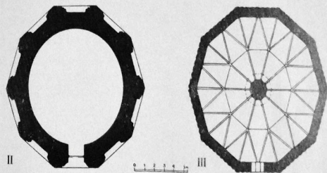
Мө'минә хатын түрбәси: I—үмүмү көрүнүшү, II—план, III—сәрдабәни планы
