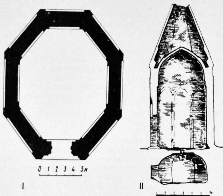
Юсиф Күсејір оғлу түрбәсі: I—план, II—кәсік, III—үмүм көрүнүшү
