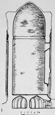
Мө'минә хатын түрбәсі: I—кәсік, II—түрбәниң јан тәрәфдән көрүнүшү
